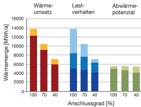
Abb. 90: Lastverhalten Ist-Zustand in Abhängigkeit des Anschlussgrades, Grundlast aus BHKW, 700 kW therm
