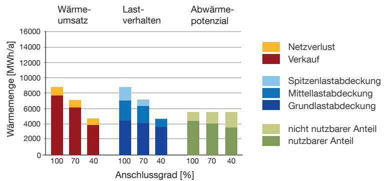
Abb. 87: Lastverhalten Zukunftsszenario in Abhängigkeit des Anschlussgrads, Grundlast aus BHKW, 700 kW therm
