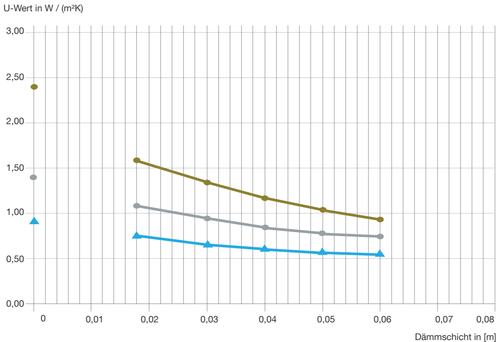
Abb. 48: U-Werte unterschiedlicher Putzstärken für Konstruktionsklasse A und B
