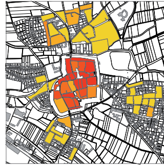
Abb. 38: Heizwärmebedarf der Wohngebäude Stadt Iphofen IST
