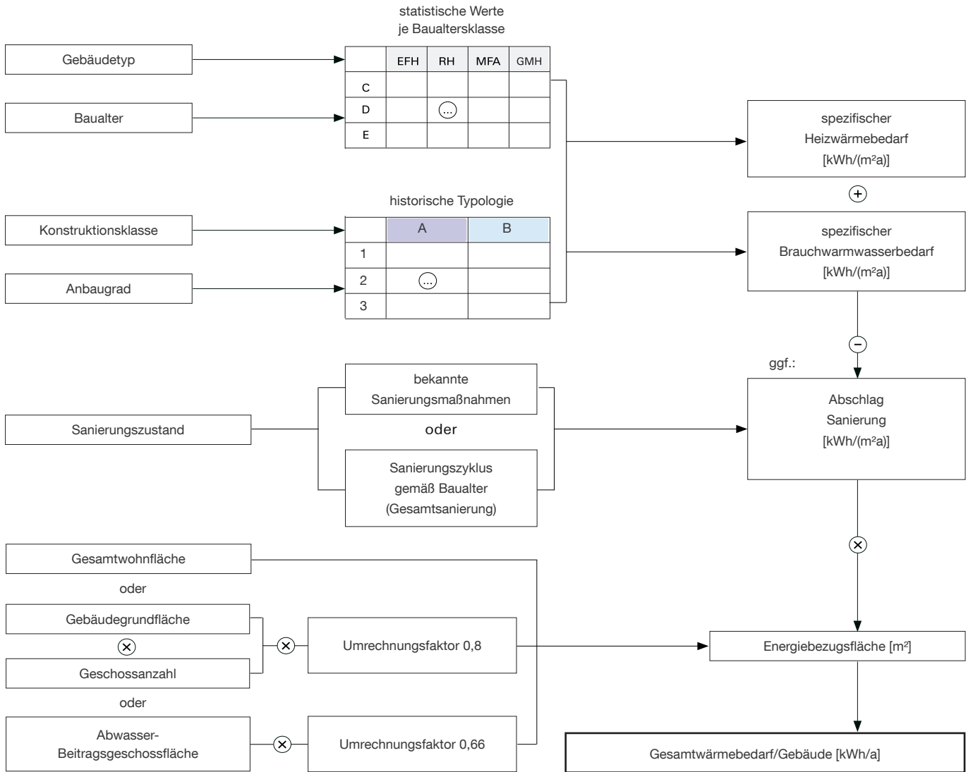
Abb. 15: Wärmebedarfsermittlung gewachsener historischer Quartiere nach IWU und HEGT modifiziert nach [Hausladen et al., 2011]
