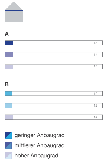
Abb. 53: Einsparpotenzial in kWh/(m²a) durch die Dämmung der Obersten Geschosdecke von 20 cm WLG 040
