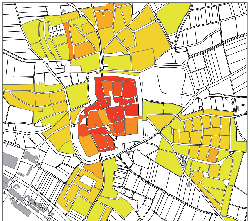
Abb. 27: Wärmebedarfsdichte der IST-Situation im Stadtbereich Iphofen
