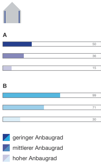
Abb. 45: Einsparpotenzial in kWh/(m²a) einer Innenwanddämmung mit 7 cm und WLG 060 für Konstruktionsklasse A und B
