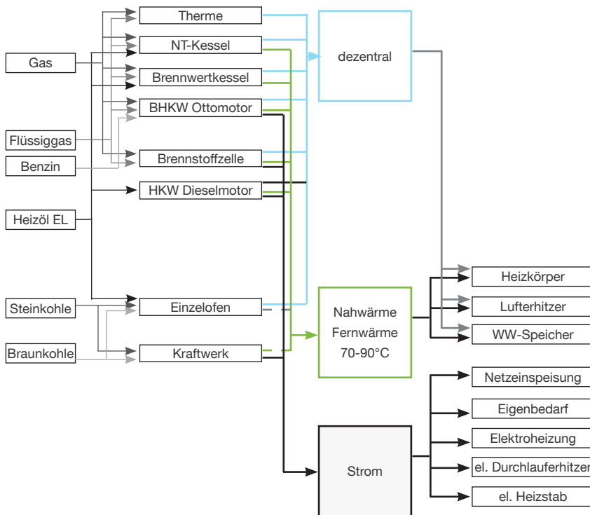
Abb. 68: Adaption von neuen und bestehenden Anlagekomponenten - fossile Energieträger
