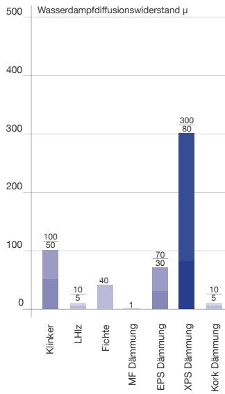
Abb. 44: Wasserdampfdiffusionswiderstand \mu unterschiedlicher Baustoffe
