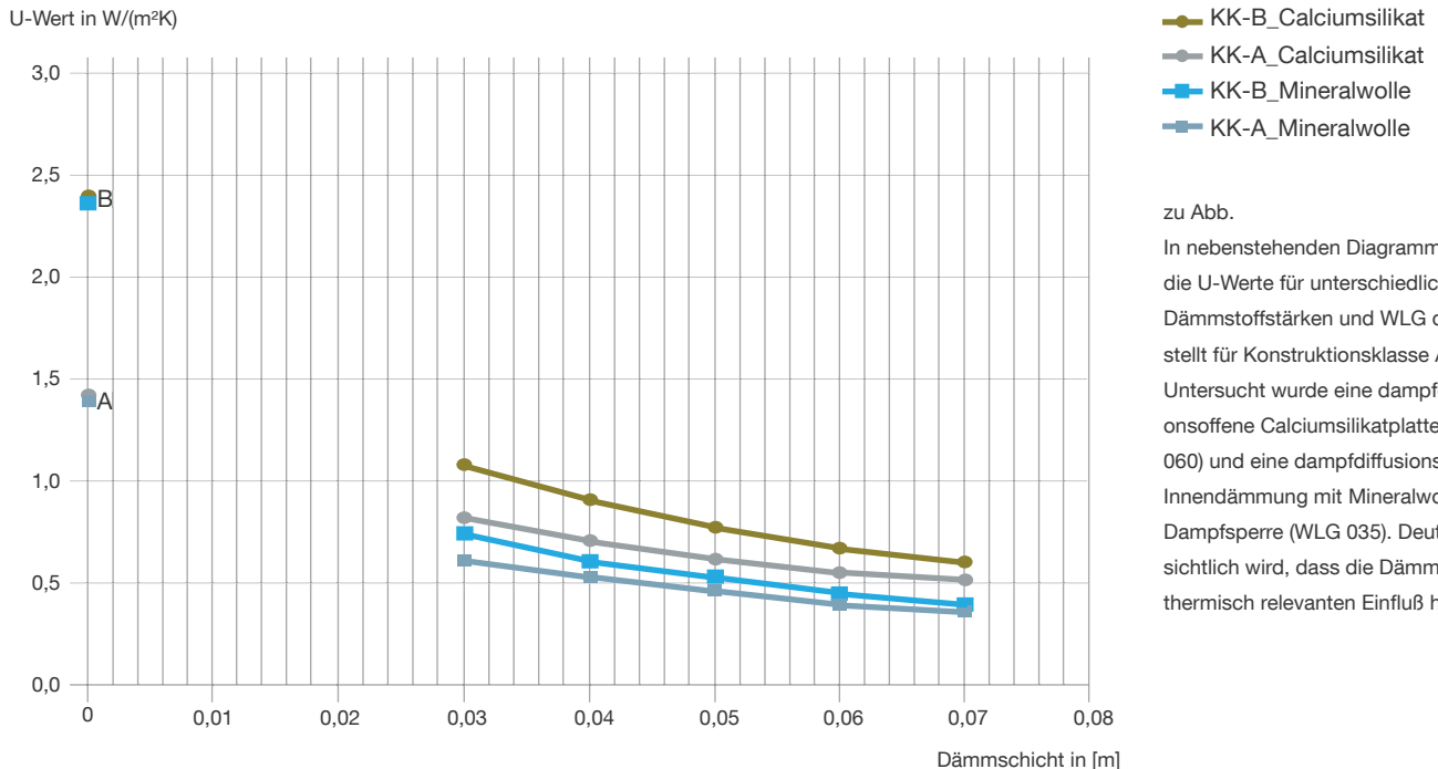
Abb. 47: U-Werte unterschiedlicher Dämmstoffstärken und WLK, für Konstruktionsklasse A und B
