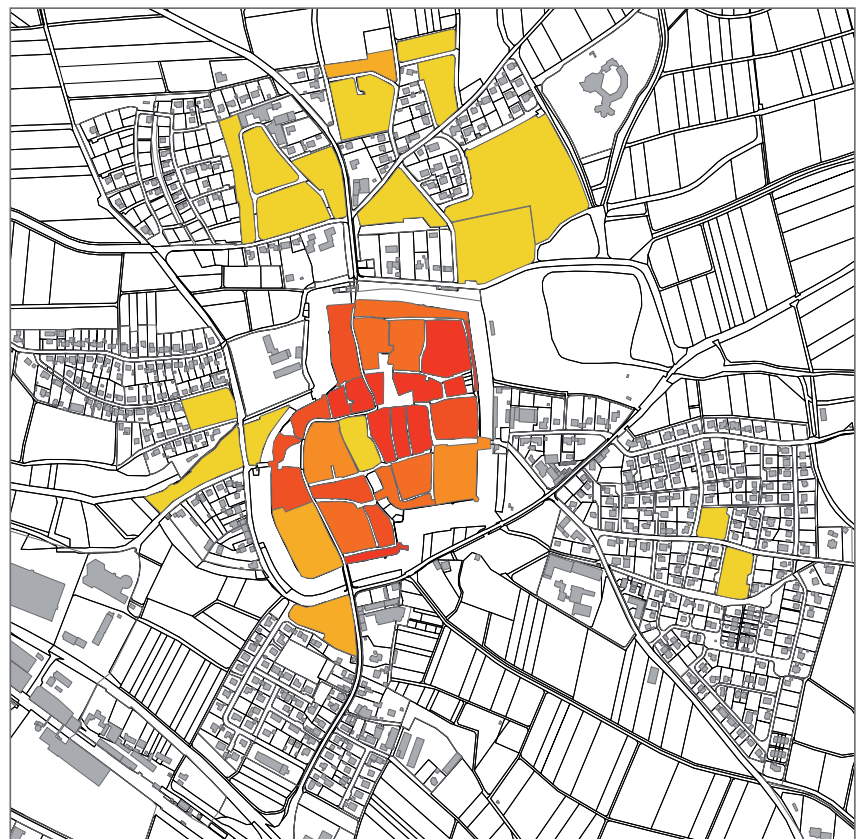
Abb. 30: Wärmebedarfsdichte Zukunft: jährliche Sanierungsrate 1,5% - Anschlussgrad 70%
