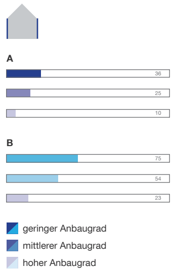
Abb. 49: Einsparpotenzial Wärmedämmputz in kWh/(m²a) (5cm WLG 090)
