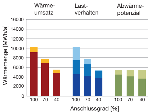
Abb. 84: Lastverhalten Ist-Zustand in Abhängigkeit des Anschlussgrads, Grundlast aus BHKW, 700 kW therm
