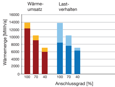
Abb. 89: Lastverhalten Ist-Zustand in Abhängigkeit des Anschlussgrads
