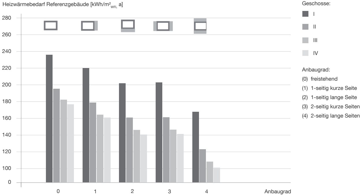
Abb. 96: Heizwärmebedarfswerte der untersuchten Gebäude der Konstruktionsklasse A in Abhängigkeit des Anbaugrads
