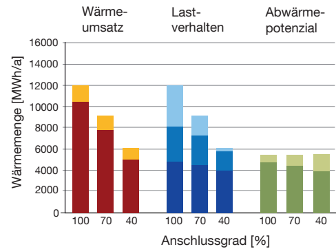
Abb. 93: Lastverhalten Zukunftszenario in Abhängigkeit des Anschlussgrades, Grundlast aus BHKW, 700 kW therm
