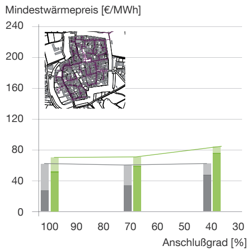
Abb. 70: Mindestwärmepreise der Altstadt Iphofen, Ist-Zustand (unten) und Zukunftsszenario bei Vollsanierung (oben) in Abhängigkeit des Anschlussgrads
