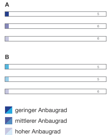
Abb. 54: Einsparpotenzial in kWh/(m 2 a) Dämmung mit 6 cm WLG 035 einer Kellerdecke U=0,8 W/m 2 K
