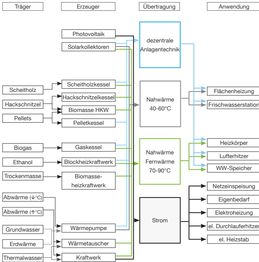
Abb. 67: Adaption von neuen und bestehenden Anlagekomponenten - erneuerbare Energieträger
