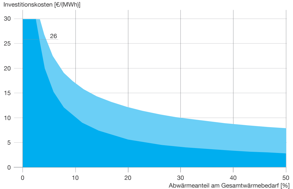
Abb. 95: Spezifische Kosten (unten) und Verbrauch (oben) in Abhängigkeit der eingespeisten Energie bezogen auf den Gesamtwärmebedarf der Netzausbauvariante "Altstadt" im IST-Zustand bei 70 % Anschlussgrad
