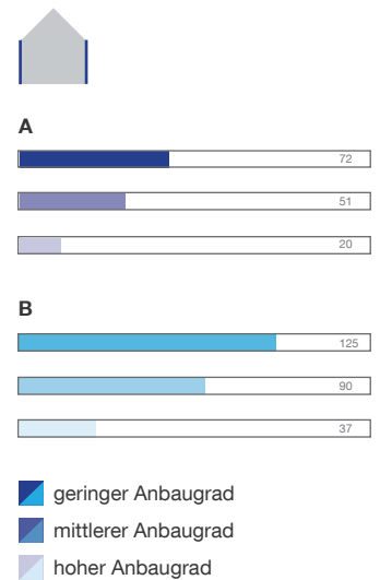
Abb. 43: Einsparpotenzial* in \text{kWh}/(\text{m}^2\text{a}) einer Außenwanddämmung mit 15 cm WLG 035 für Konstruktionsklasse A und B
