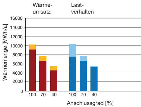
Abb. 83: Lastverhalten Ist-Zustand in Abhängigkeit des Anschlussgrads
