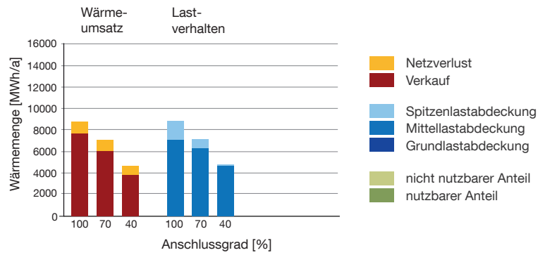
Abb. 86: Lastverhalten Zukunftsszenario in Abhängigkeit des Anschlussgrads
