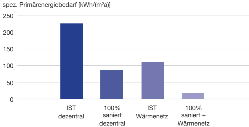
Abb. 77: Spezifischer Primärenergiebedarf der Altstadt Iphofen für historische und nicht-historische Gebäude im Ist-Zustand und in den Zukunftsszenarien für dezentrale und zentrale Wärmeversorgung
